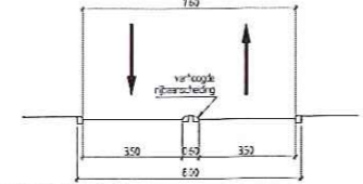
Principeprofiel 2-2 schaal 1:100
