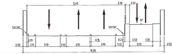
Principeprofiel 1-1 schaal 1:100
