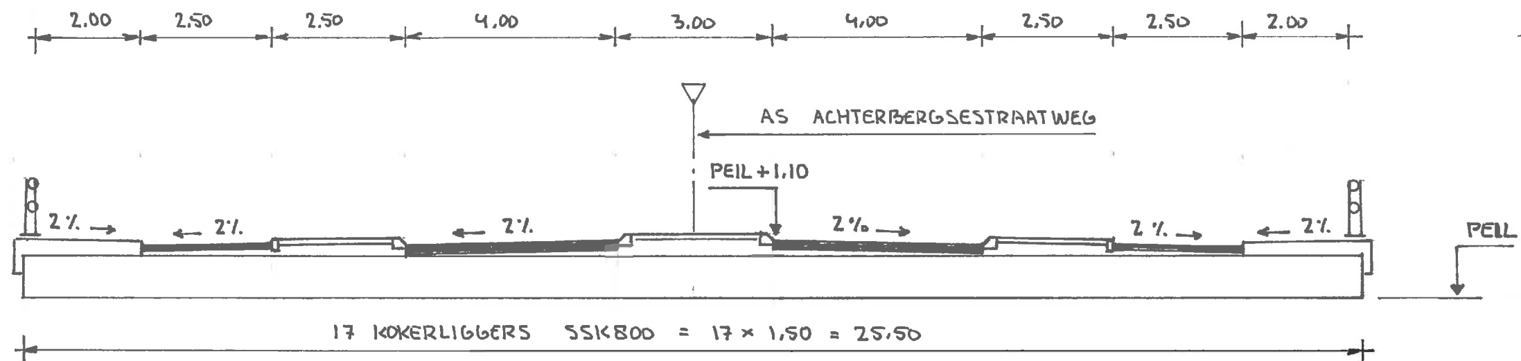
DWARSDOORSNEDEN VIADUCT ACHTERBERGSESTRAATWEG OVER N233
